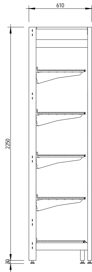
3 End Elevation 1 : 20
