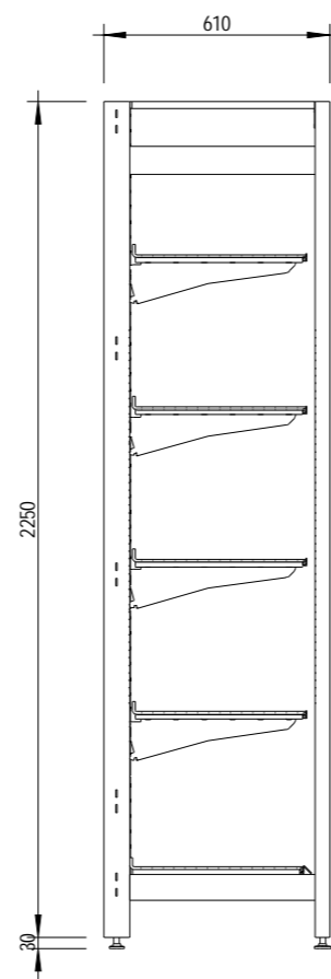
3 End Elevation 1 : 20
