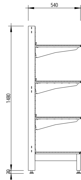
3 End Elevation 1 : 20
