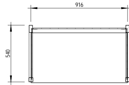
1 Plan 1 : 20
