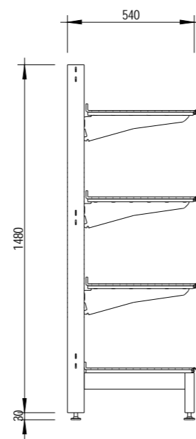
3 End Elevation 1 : 20
