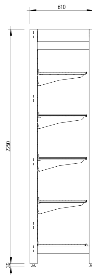
3 End Elevation 1 : 20
