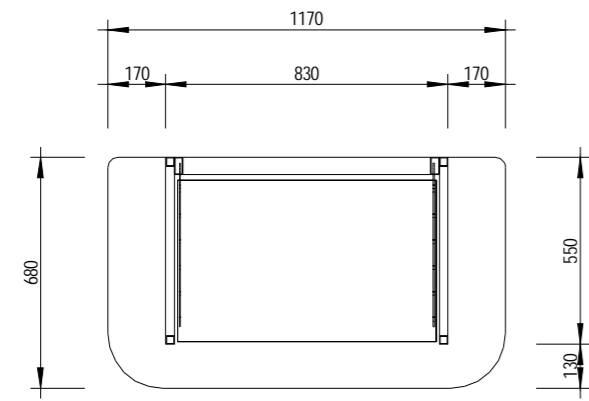
1 Plan 1 : 20
