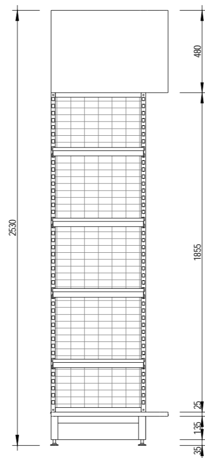
3 End Elevation 1 : 20
