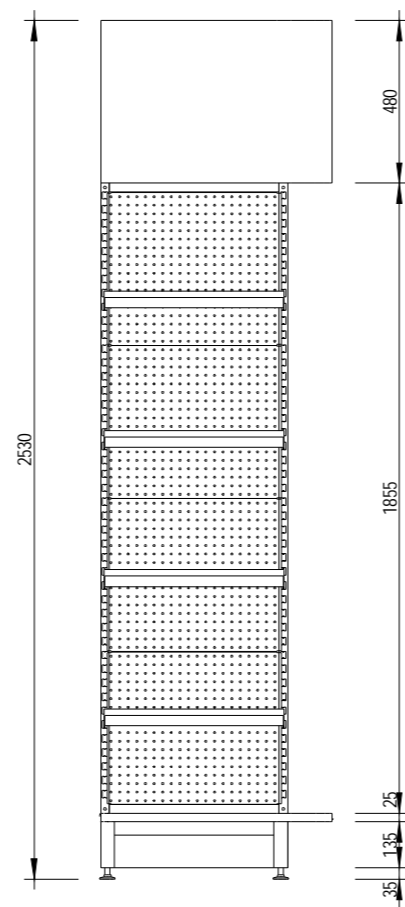
3 End Elevation 1 : 20
