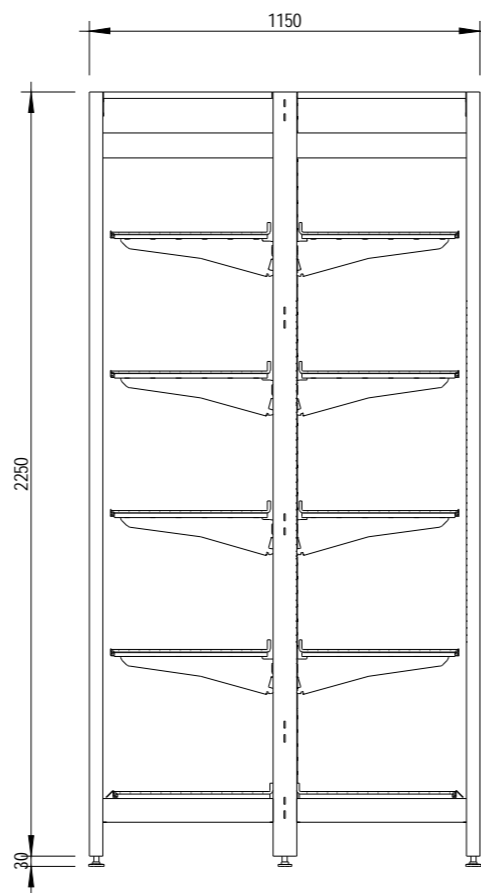
3 End Elevation 1 : 20
